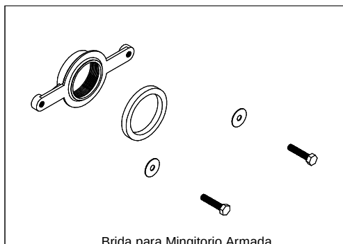
SX-SF-645 Brida para Mingitorio Armada Urinal Flange Armed
